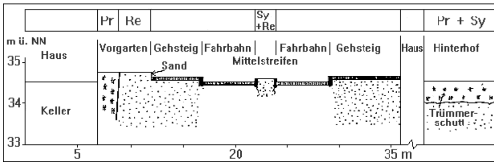
Abb. 10: Lockersyrosem + Regosol + Pararendzina (Böden der Innenstadt auf Aufschüttungen)
